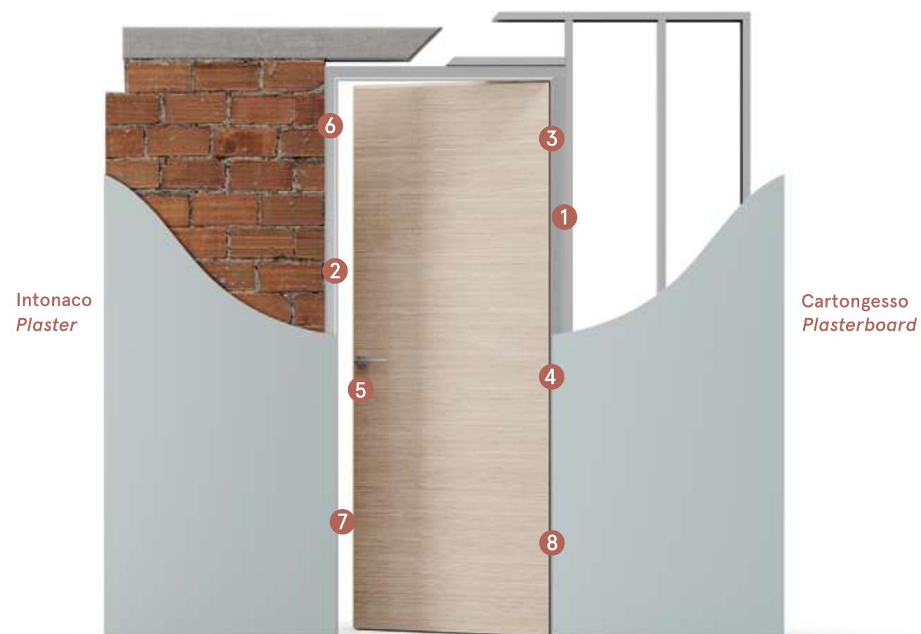
Porta battente Filo Muro Flush hinged door system
